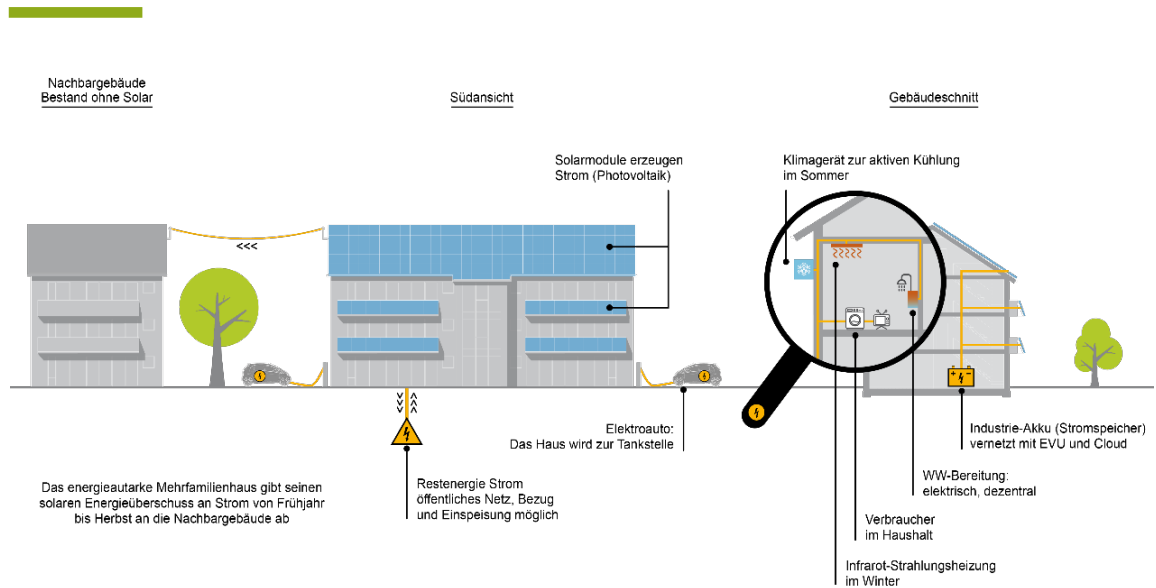
➤ Abb. 2: Prinzip der Energieautarkie, PV-Module auf Dächern, an Balkonbrüstung und Fassade. Elektrische Wärme- und Kälteversorgung durch wartungsfreie Infrarotheizung und Kühlung, sowie dezentrale Warmwasserbereitung. Das E-Auto gehört zum Gebäude – das Haus wird zur Tankstelle für die Mieter.
